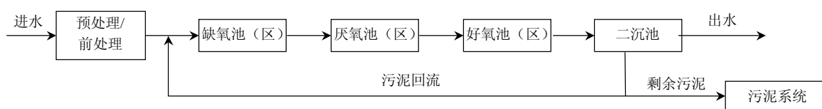
图 A.4 RAAO 工艺流程图
