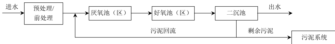
图 1 厌氧好氧工艺流程图
