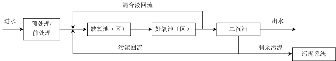
图 2 缺氧好氧工艺流程图
