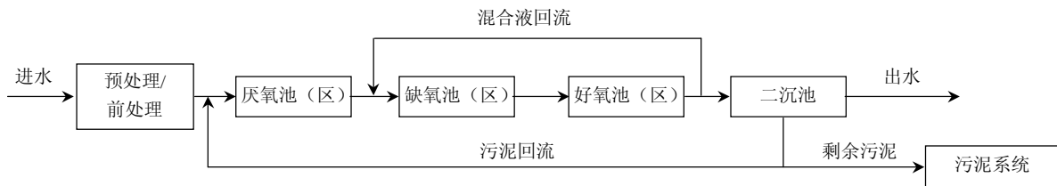
图 3 厌氧缺氧好氧工艺流程图
